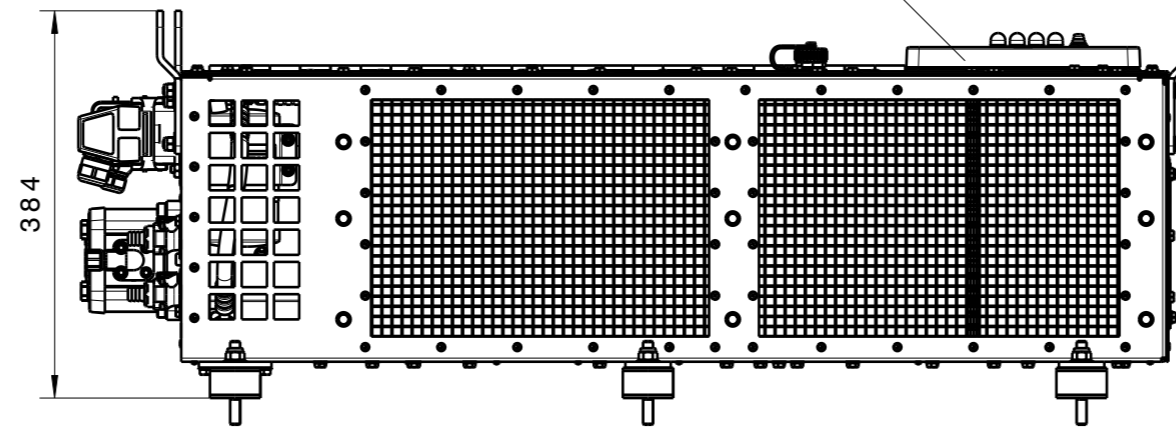
Vorderansicht
