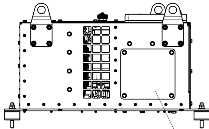
Seitenansicht rechts
