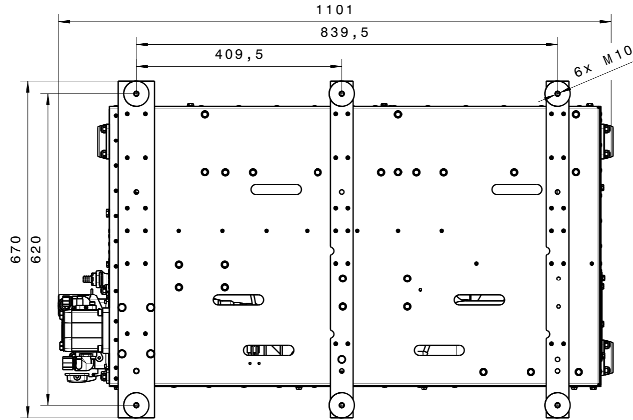
Untersicht
