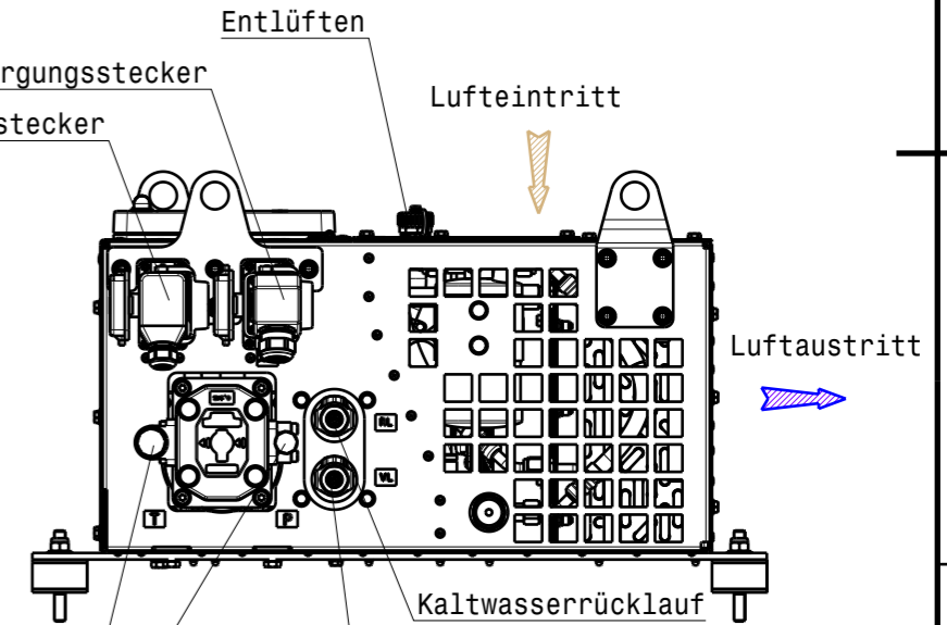
Seitenansicht links
